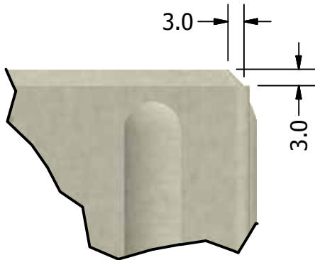
CHAMFER 3 3mm x 3mm (45°)
