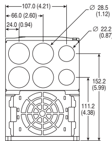
C Frame - 22-JBAC
